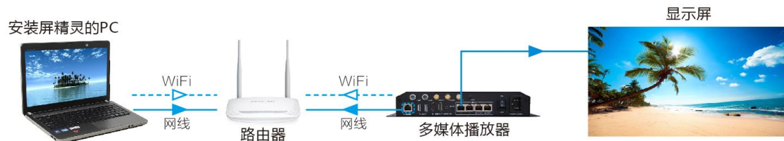
图2-3 局域网连接
