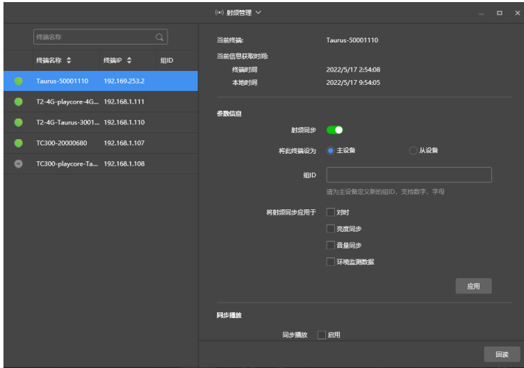
图4-56 射频配置
