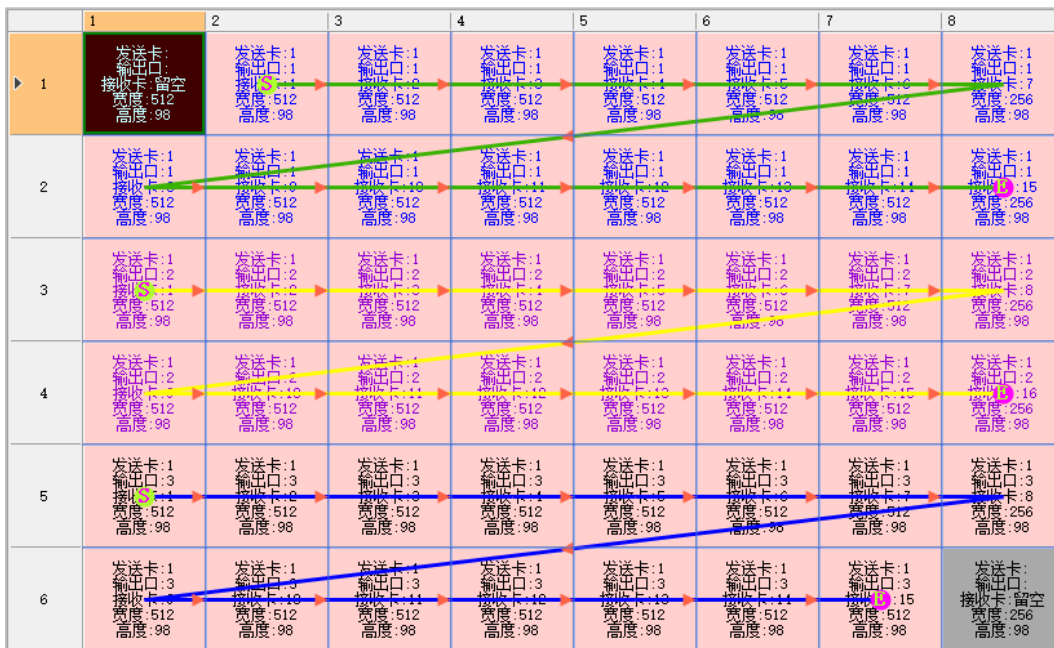
图3-4 超长屏接收卡留空
