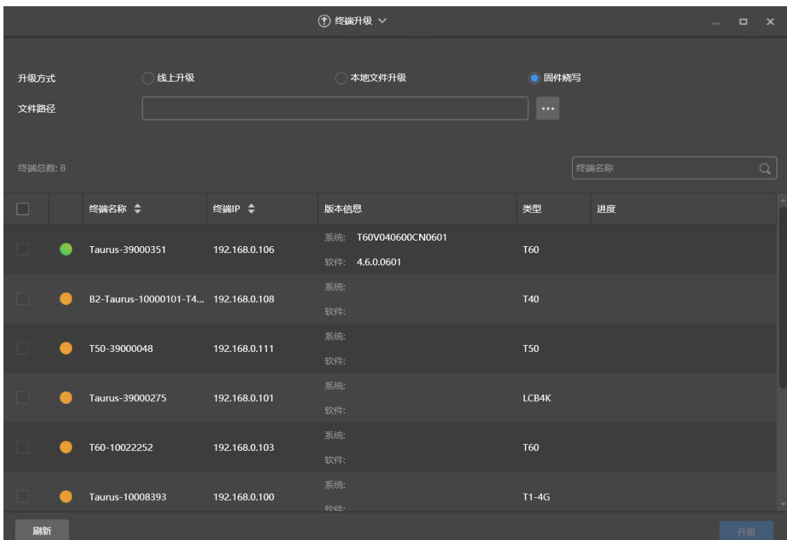
图4-52 固件烧写
